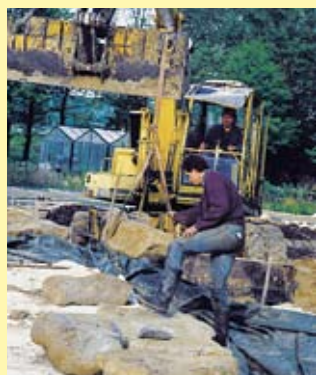
Der Einbau von tonnenschweren Trittsteinen über der Folie erfordert Vlies900 oder Verbundmatte als Schutzlage.
